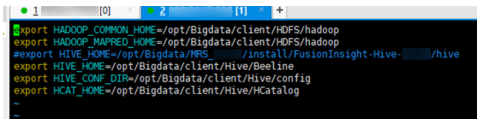
图 27-3 设置 Sqoop 的环境变量
