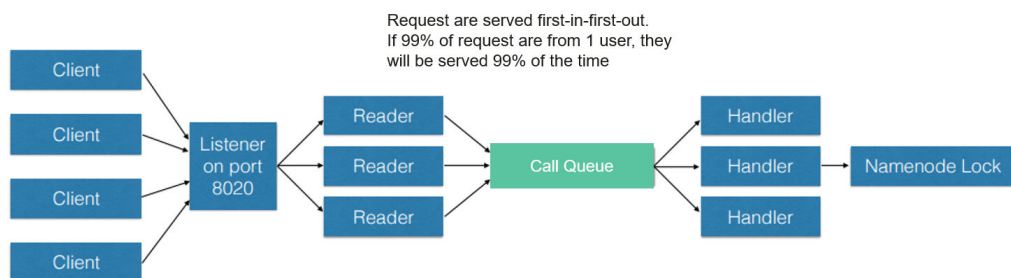
图 9-9 基于 FIFO 调用队列的 NameNode 请求处理
