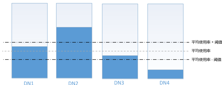
图 9-6 执行均衡操作前 DataNode 的磁盘使用率
