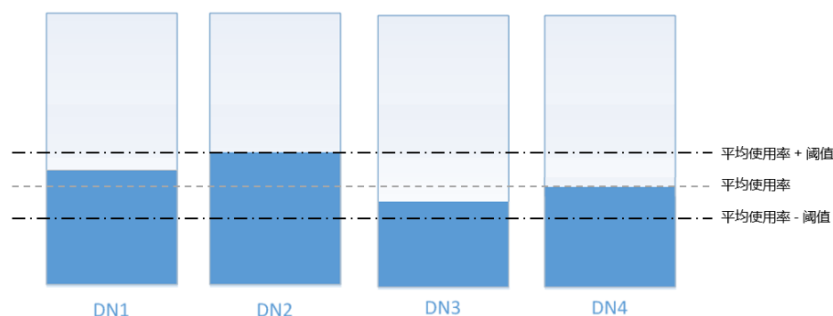
图 9-7 执行均衡操作后 DataNode 的磁盘使用率
