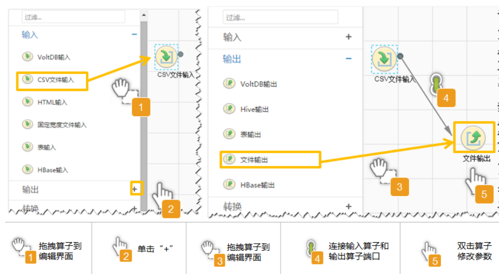
图 17-54 算子操作方法示意
