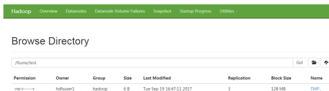
图 7-10 查看 HDFS 目录和文件
